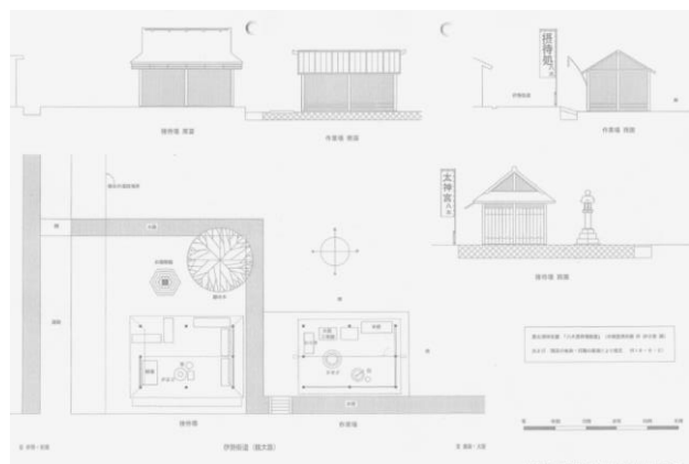
八木せんたい場図面
