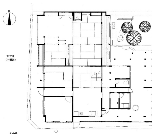
東の平田家 1 階平面図
