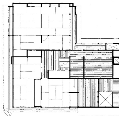
東の平田家 2 階平面図
